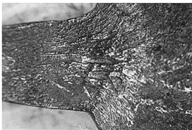
Fig. 7: Estructura micrográfica (fibrado longitudinal).
