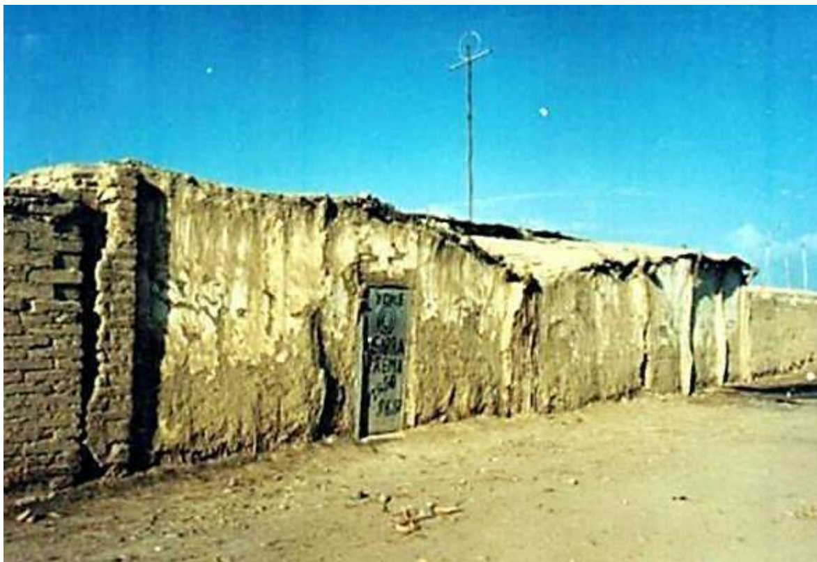
Figura 8. Casa tradicional elaborada con caña, madera de algarrobo y tierra.
