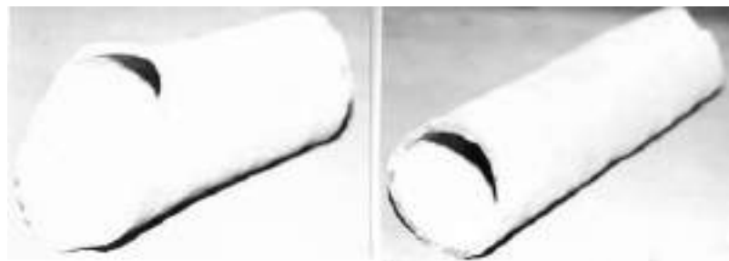
Fig. 5. El análisis del recubrimiento, corroborado por determinaciones de difracción de rayos X, determinó que está formado por cloruros y sulfuros principalmente de plomo, con la presencia de silicatos de calcio y potasio (Pifferetti 1997a).
