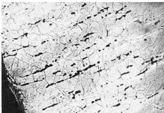
Fig. 8: Estructura micrográfica (inclusiones alargadas en sentido de la deformación).
